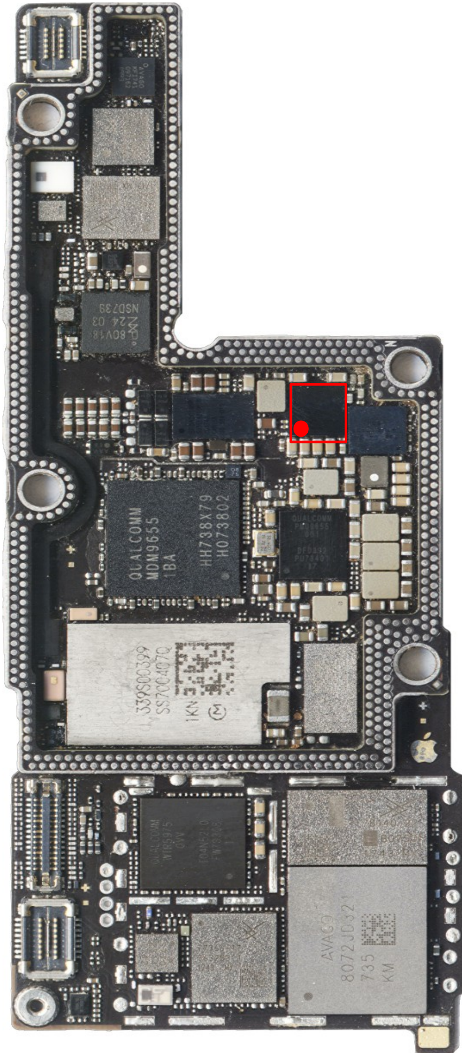
iPhoneX U5000听筒+扬声器二合一放大管对地阻值图
